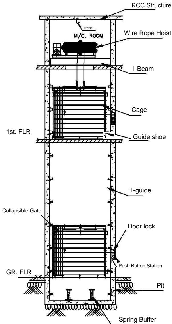
ELEVATION
